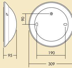
Größe 1 Ø 309 mm
