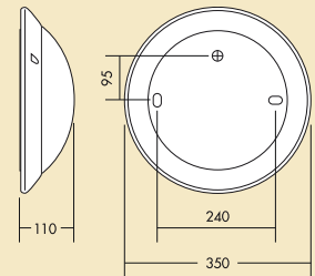
Größe 2 Ø 350 mm
